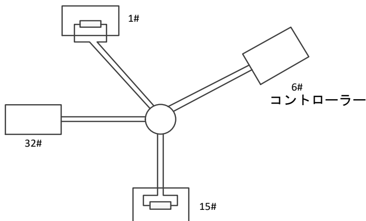
図 A.5.3 スター型接続
