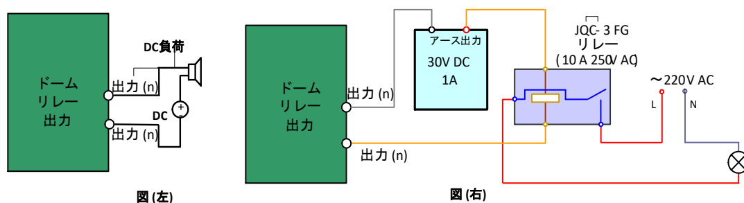
図 A.9.1 アラーム出力接続
