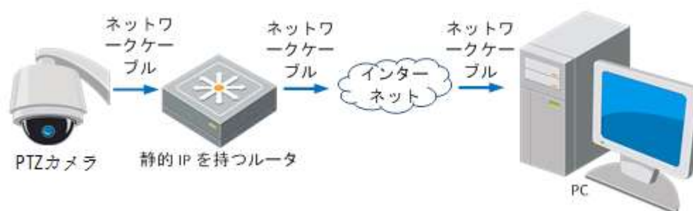
図 2-11 静的 IP を持つルータを経由した PTZ カメラへのアクセス
