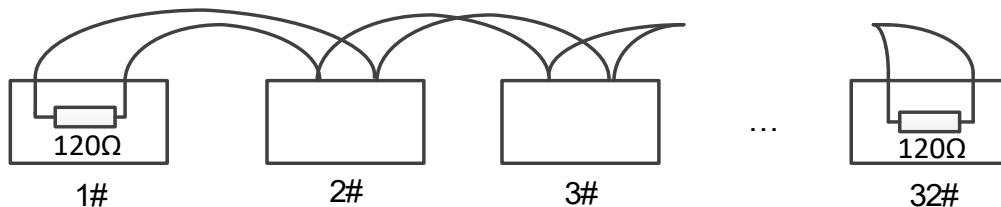
図 A.5.1 RS485 接続 1
