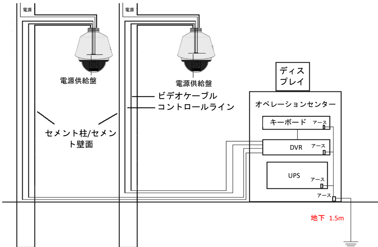
図 A.2.2 セメント柱/セメント壁面設置時のアース
