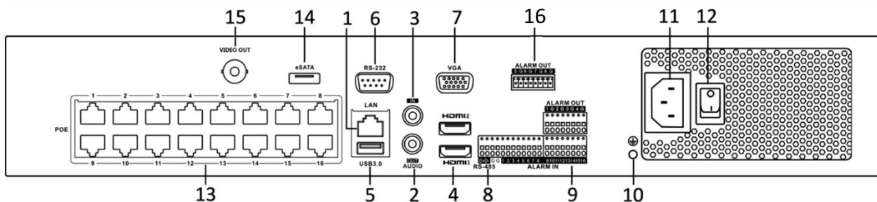
図 1-13 DS-7700NI-I4/16P(B)シリーズ
